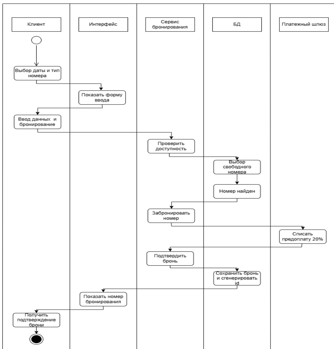
Рисунок 6 — Диаграмма деятельности
