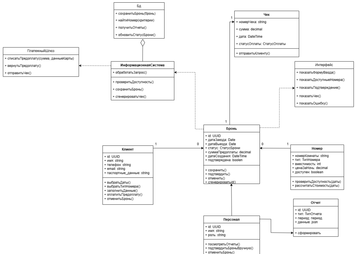
Рисунок 8 — Диаграмма классов
