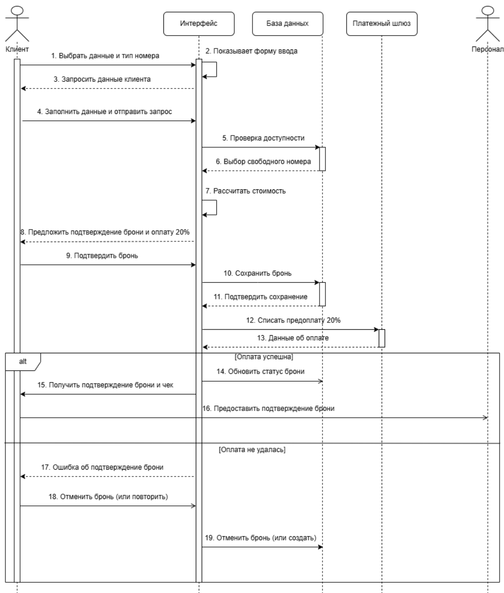
Рисунок 7 — Диаграмма последовательности
